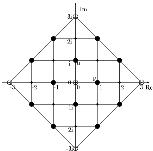
Рис. 2. Соотношение ключевых решений, описывающих состояния ядеров в сильных взаимодействиях
