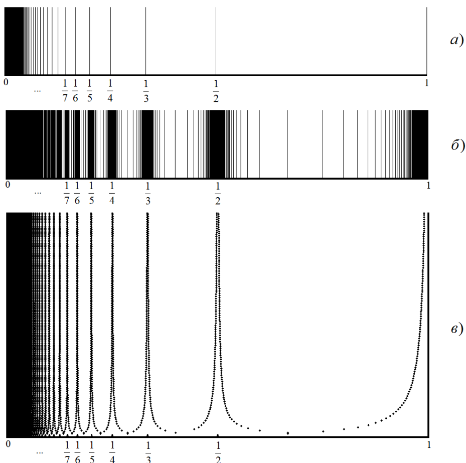
Рис. 1. Распределения рациональных a – b чисел
