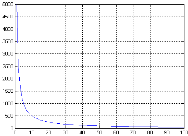
Рис. 2. Мощность классов эквивалентности для L = 5000 : ось X : значения q(1) ; ось Y : мощность классов эквивалентности
