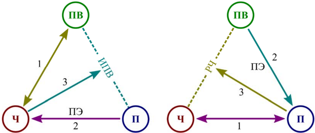
Рис. 4. Схема, демонстрирующая роль принципа эквивалентности (ПЭ) в ОТО (слева) и принципа полного поглощения в реляционной теории (справа)
