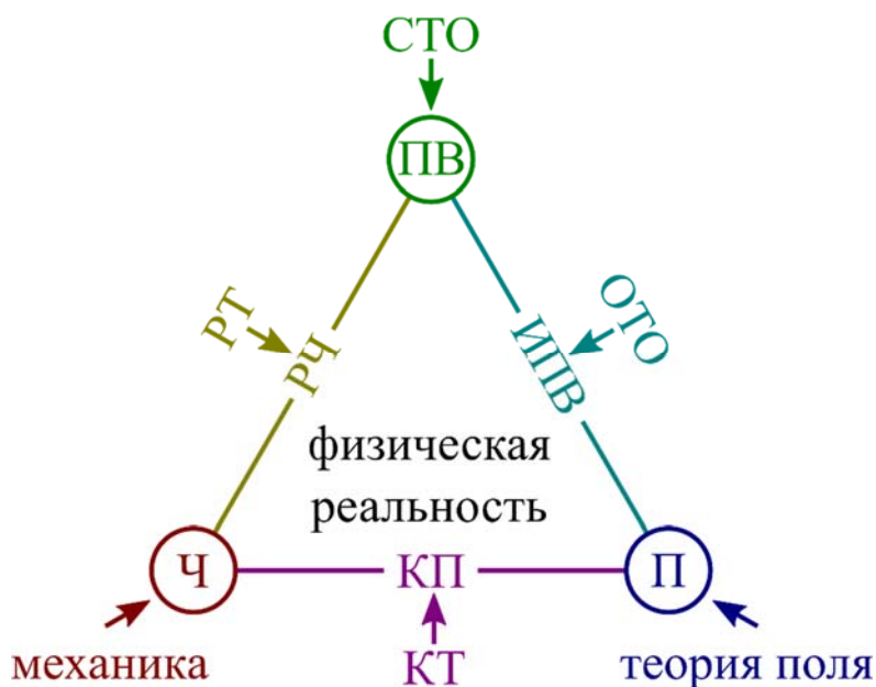
Рис. 1. Схематическое изображение основных категорий теоретической физики и соответствующих способов описания физической реальности:
