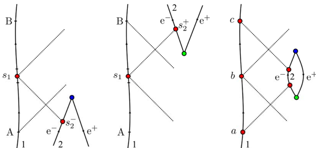
Рис. 6. Взаимодействие частицы 1 с частицей 2, входящей в пару частица–античастица
