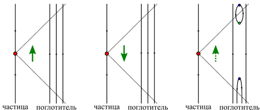
Рис. 7. Взаимодействие выделенной частицы с поглотителем. Стрелка указывает направление стрелы времени
