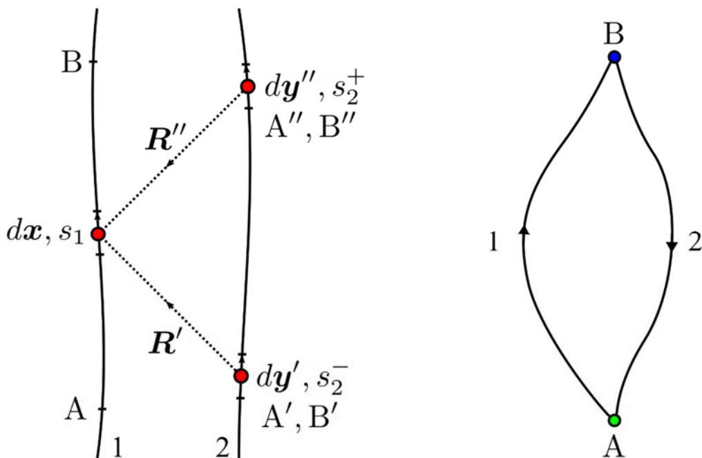
Рис 5. Мировые линии двух взаимодействующих частиц 1 и 2 (слева).
