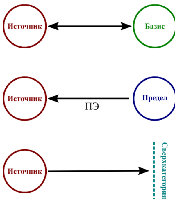
Рис. 3. Схема, поясняющая роль принципа эквивалентности (ПЭ) и его аналогов в дуалистических теориях
